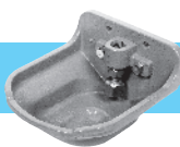
FK-11型 ボール式 (種豚用) 鋳物 幅169×高さ107×奥行188mm
