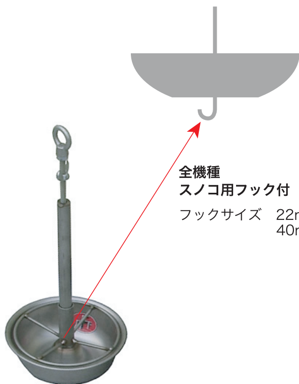
70001 S200-4型(4頭口) 容量 15kg 丸径200×H490×D65mm
